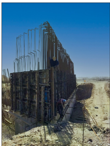
پروژه احداث تقاطع‌های غیرهمسطح فاز ۴ شبکه ریلی منطقه گل گهر پیمانکار: شرکت نکین کهرخاورمیانه هدف اجرای پروژه: تامین دسترسی‌های سایت‌های غربی منطقه گل گهر اعتبار پروژه: ۶۰۰ میلیارد ریال مشاور: شرکت رهنمای شرق راه میزان پیشرفت: ۲۰ درصد
